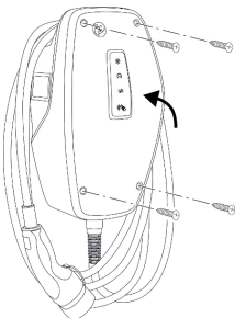
Fig. 17: Chiusura del prodotto
