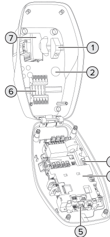
Fig. 3 : Vue de l'intérieur
