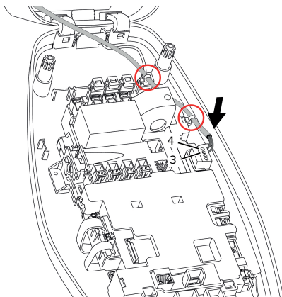
Abb. 15: Anschluss Downgrade-Eingang
