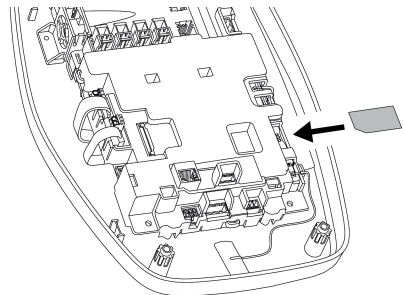
Afb. 11: SIM-kaart plaatsen
