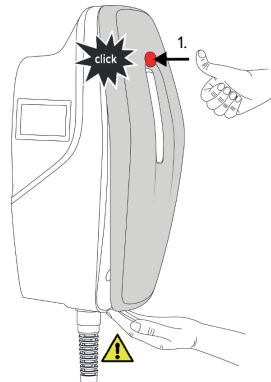
Fig. 19: Montaggio della cover anteriore - 1
