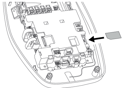
Fig. 11: Inserimento della scheda SIM
