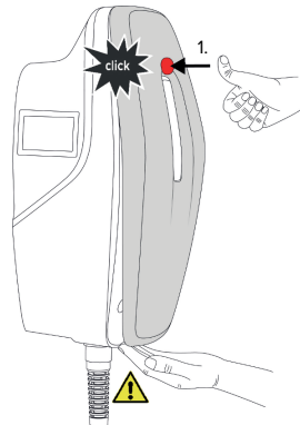
Afb. 19: Frontcover aanbrengen - 1
