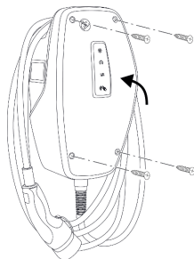
Fig. 17 : Fermeture du produit
