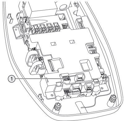
Afb. 13: Ethernetaansluiting
