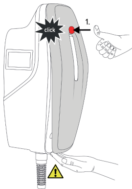
Fig. 19 : Monter le cache frontal - 1
