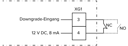
Abb. 16: Prinzipschaltbild: Anschluss eines externen Schaltkontakts (Standard-Einstellung: NO)
