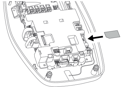
Abb. 11: SIM-Karte einsetzen
