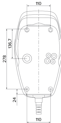
Fig. 6: Dimensioni dei fori [mm]
